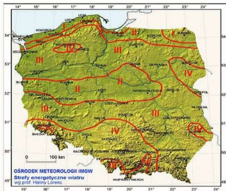
Ryc. 9 Strefy energetyczne warunków wiatrowych w Polsce wg. H. Lorenc
