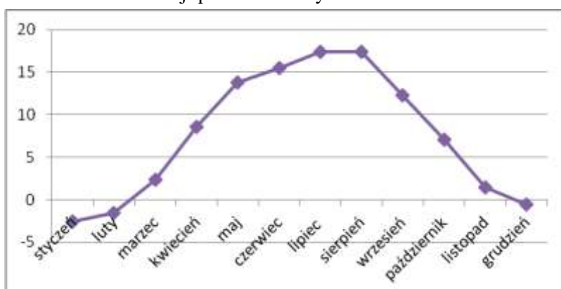
Ryc. 5 Średnie temperatury w miesiącu, w gminie Zawidz
