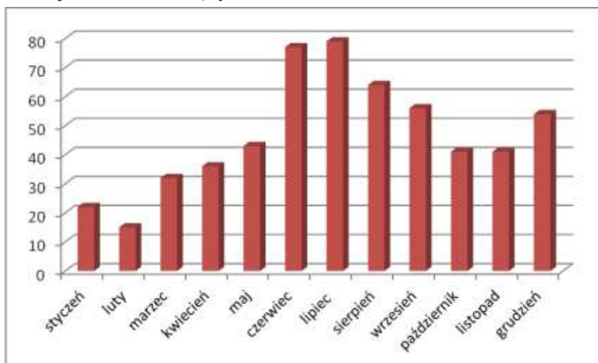
Ryc. 6 Średnie sumy opadów w gminie Zawidz
